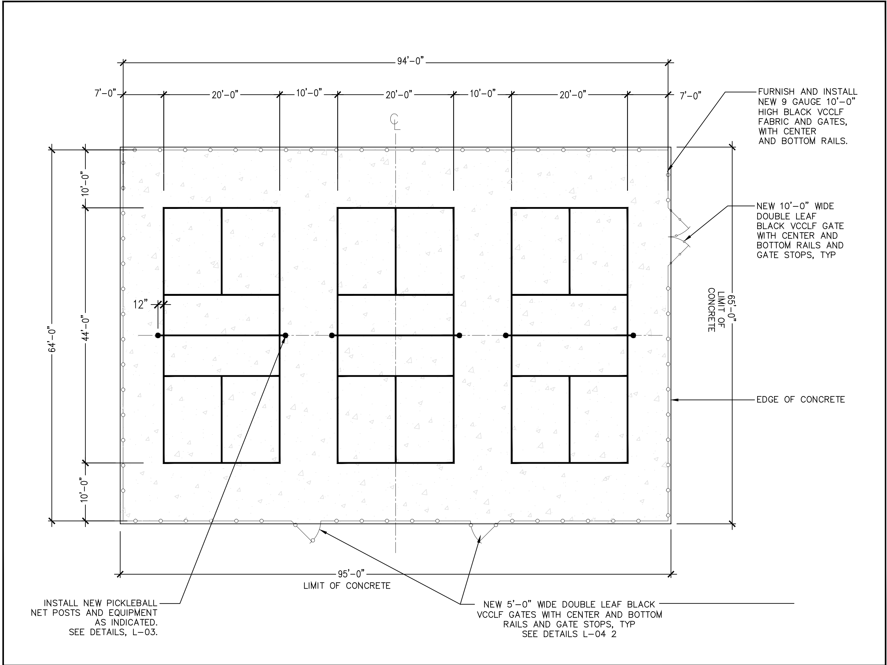
1B LAYOUT PLAN SCALE: 1" = 10'-0"
