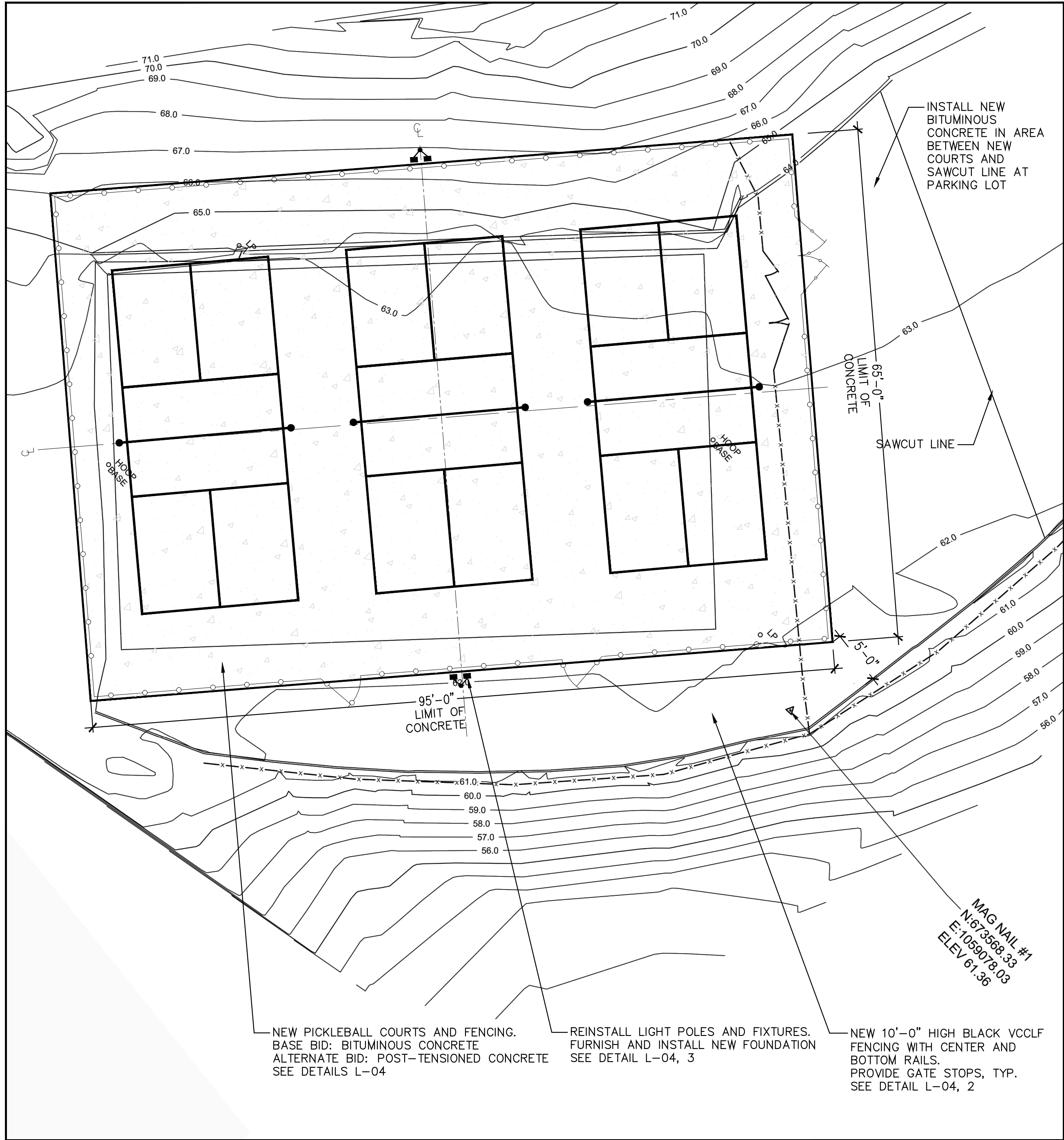
1A LAYOUT PLAN SCALE: 1" = 10'-0"
